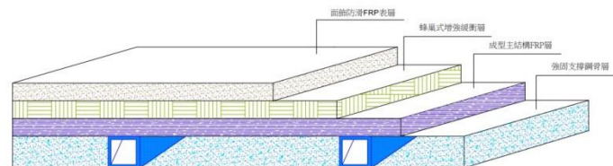
覆合防水底盤結構示意圖
